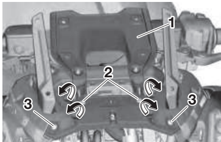
1. Cubierta interior 2. Fijación rápida 3. Tornillo
